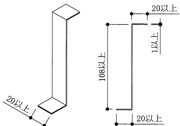
支持金具A-①
