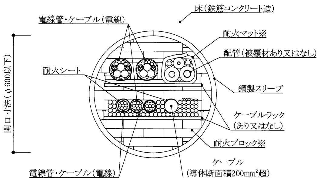
平面図(円形の一例)
