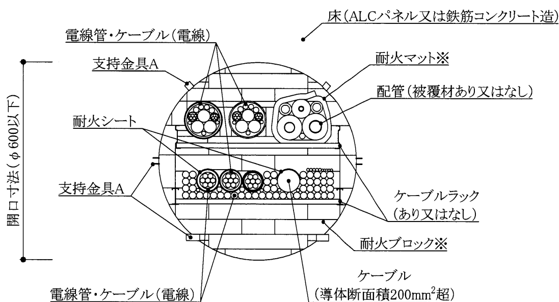
平面図(円形の一例)
