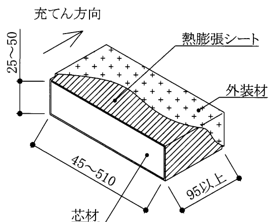
耐火ブロック詳細図の一例
