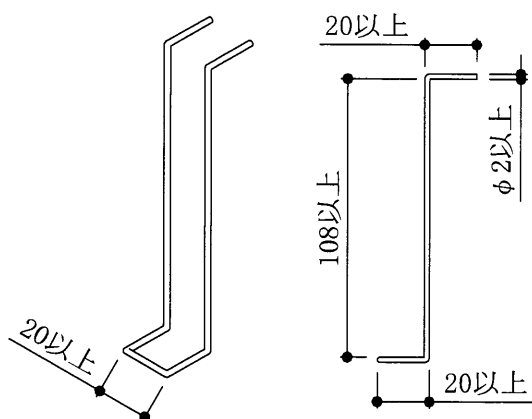
支持金具A-②
