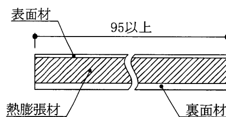
耐火シート断面図の一例
