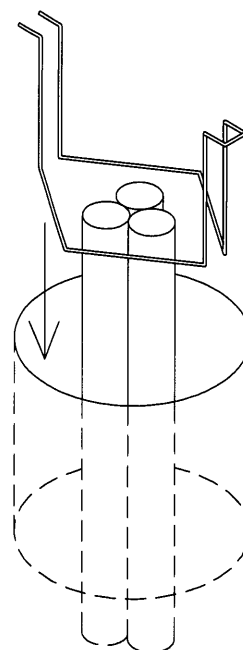
支持金具A-②(円形開口用)の一例
