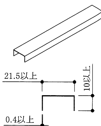
支持金具B-②
